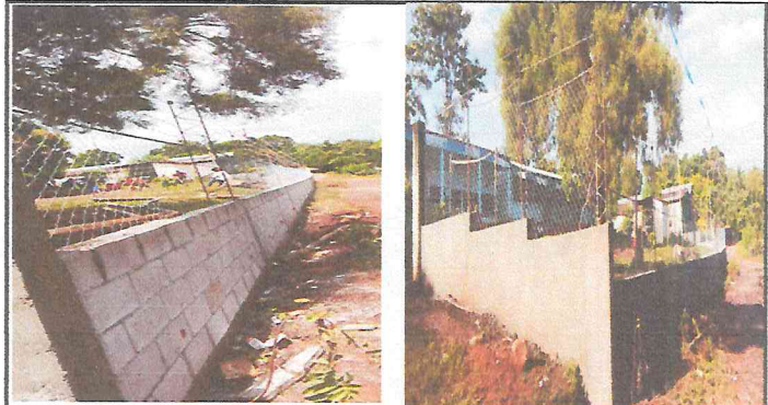
Foto 4: Finalización de la circulación y repello o cernido del área perimetral de la escuela
